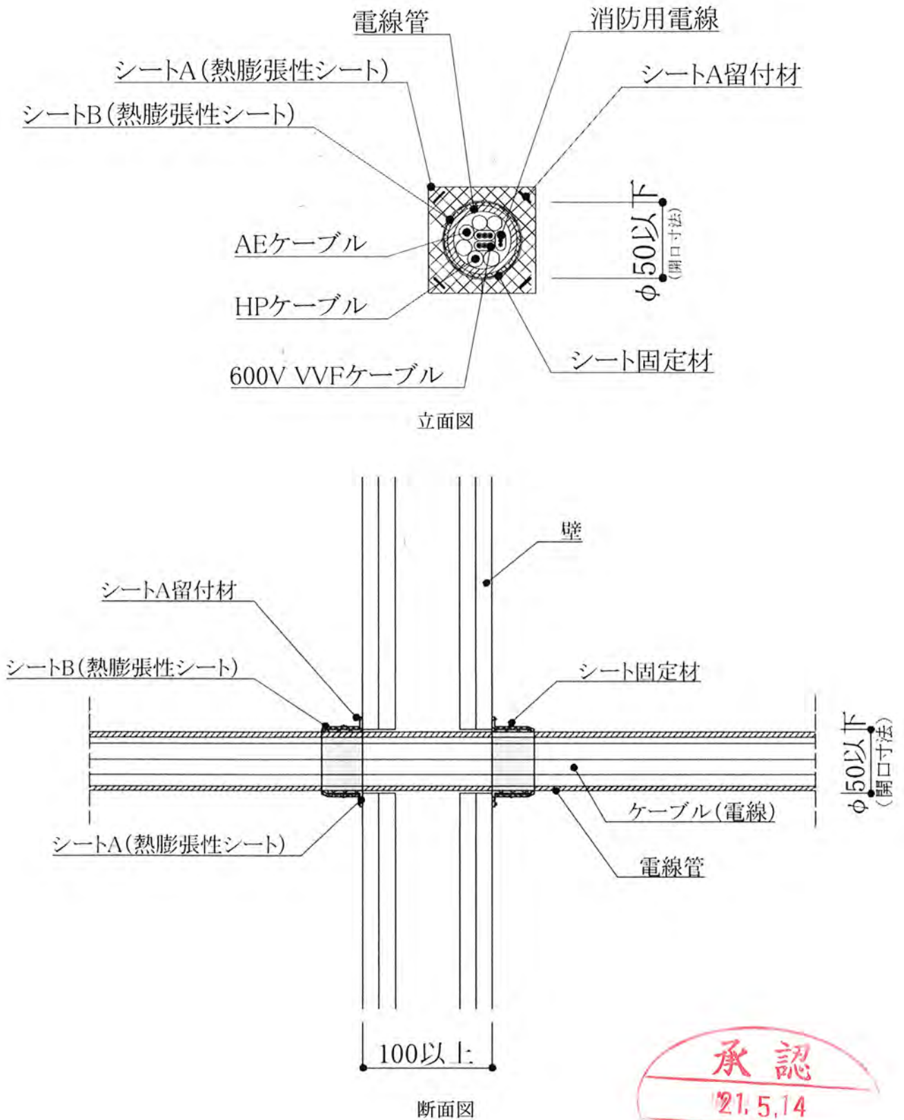
図2 施工図例
