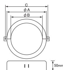
押さえ金具
