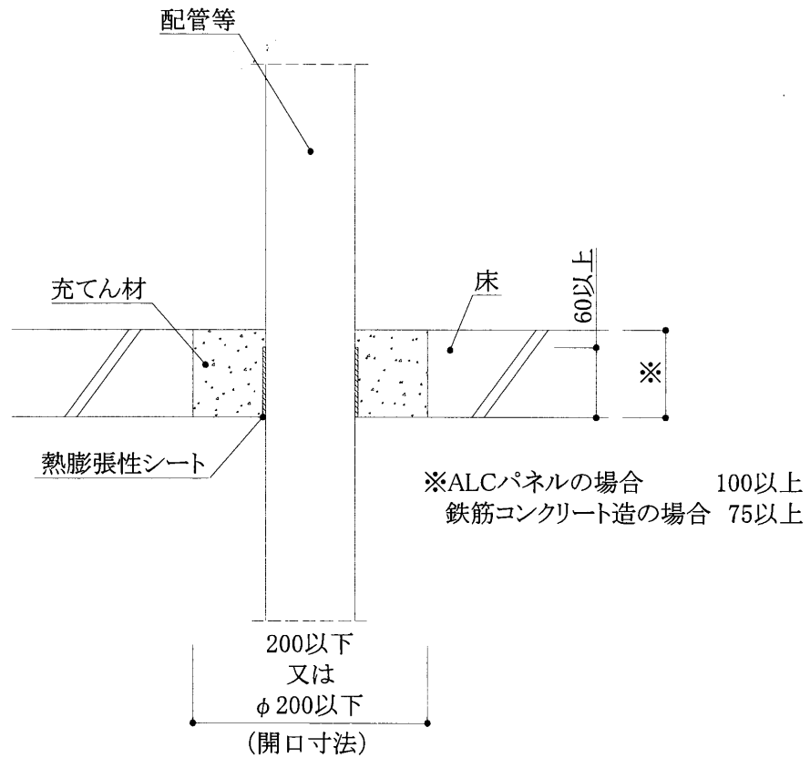
断面図
