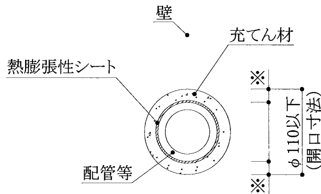
立面図(円形の場合)
