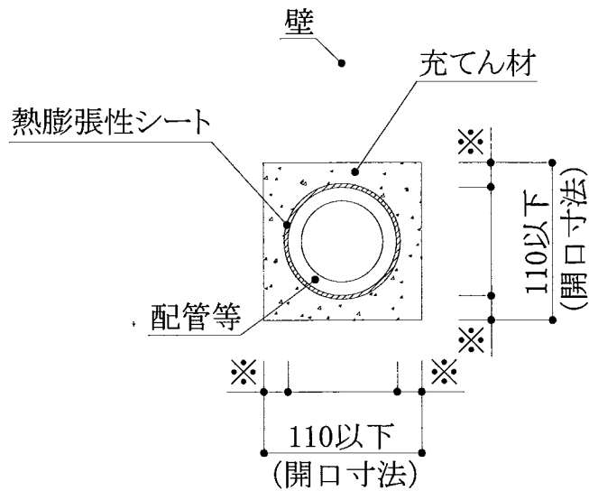
立面図(矩形の場合)
