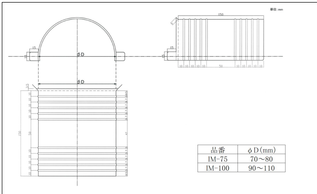
図-1 寸法図(IM-75、100)
