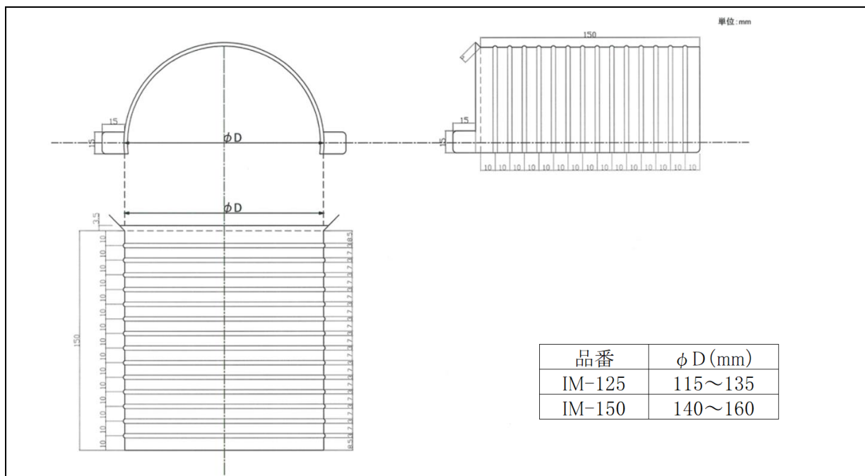
図-2 寸法図(IM-125、150)
