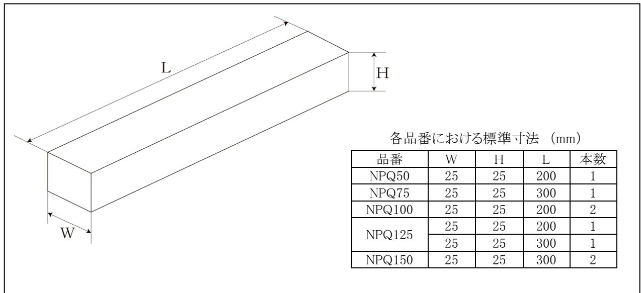
図-3 バックアップ材概略図
