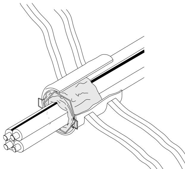
施工完成図
