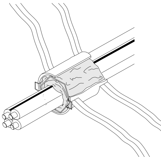
施工完成図
