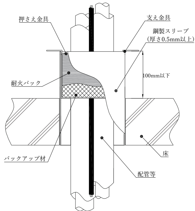
施工断面図
