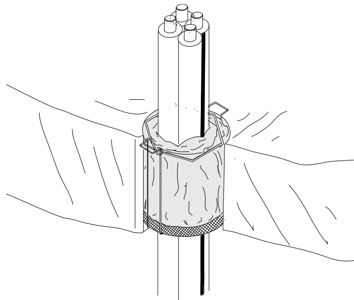
施工完成図
