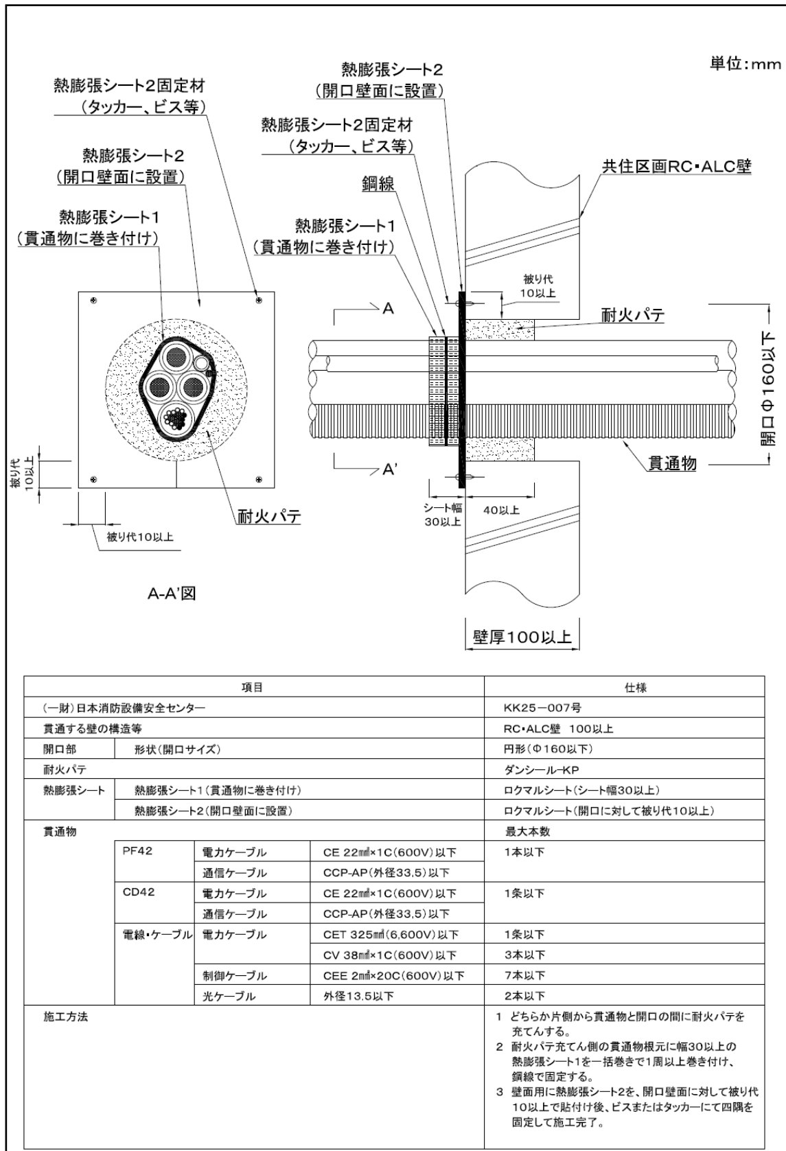
図-4-2 KK25-007号工法(共住区画RC・ALC壁)標準施工図
