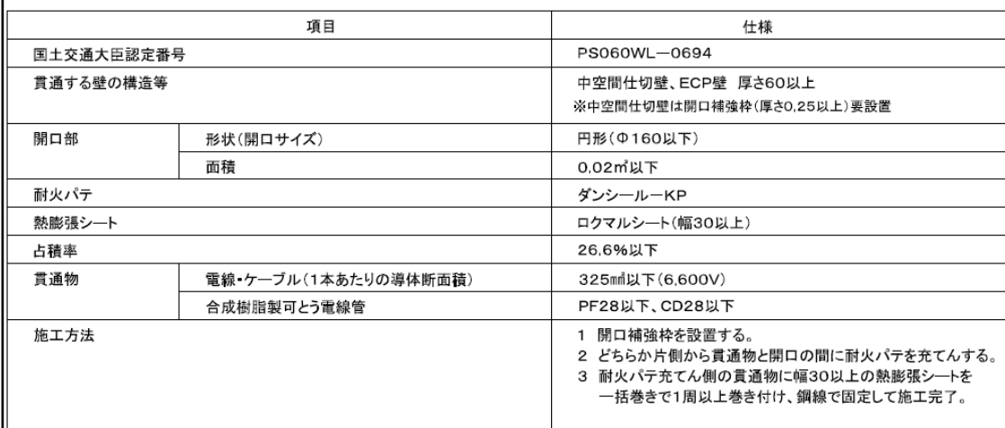
図-2 PS060WL-0694 工法(中空間仕切壁)標準施工図
