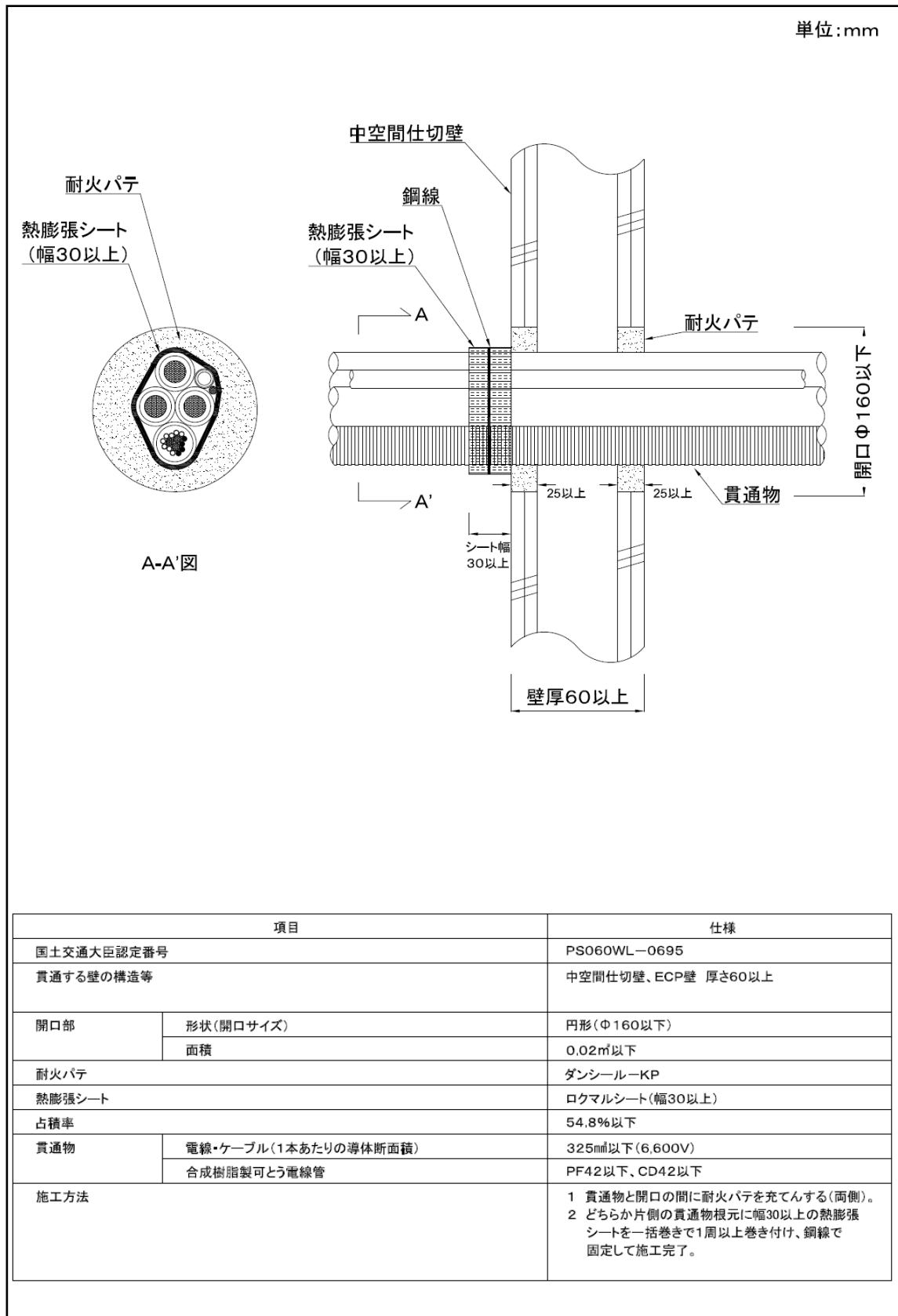
図-1 PS060WL-0695 工法(中空間仕切壁)標準施工図
