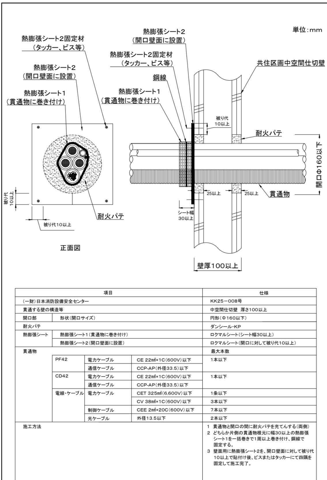
図-5 KK25-008 号工法(共住区画中空間仕切壁)標準施工図
