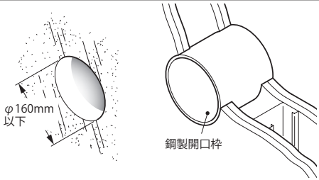
ダンシール-KP充填量(1箇所あたりの目安)
