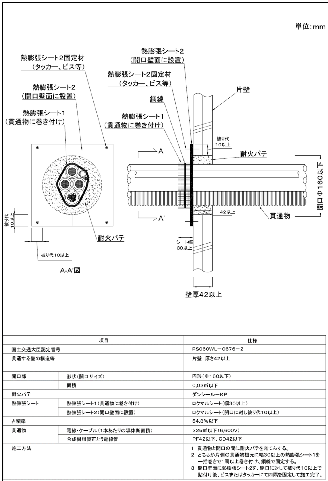
図-5 PS060WL-0676-2 工法(片壁)標準施工図
