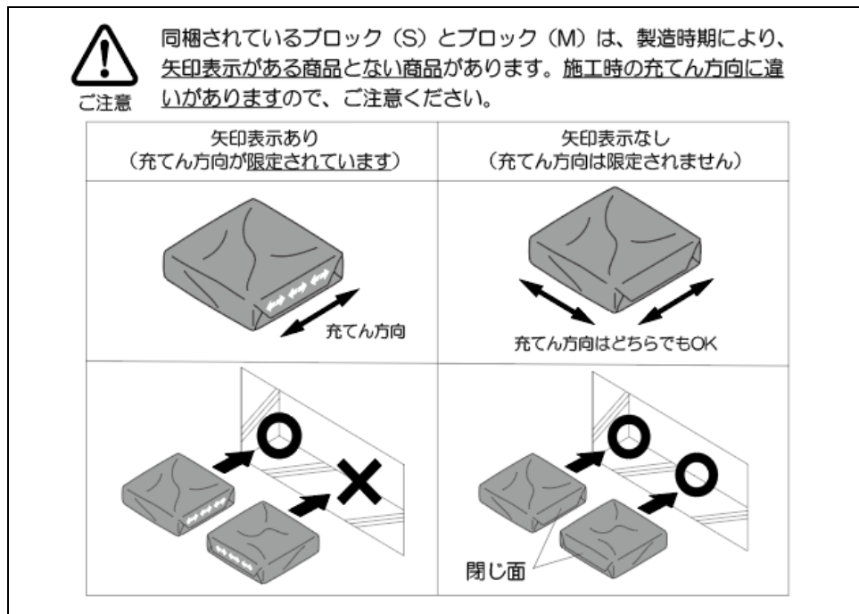
図-2 矢印表示の注意書き
