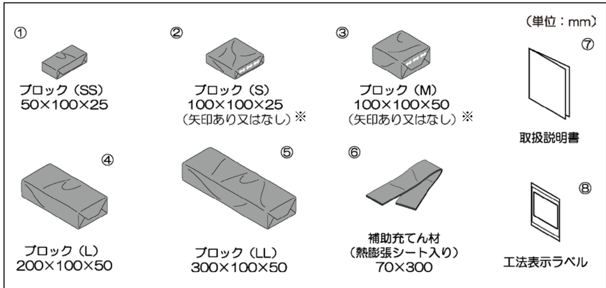
図-1 キット品構成材料一覧
