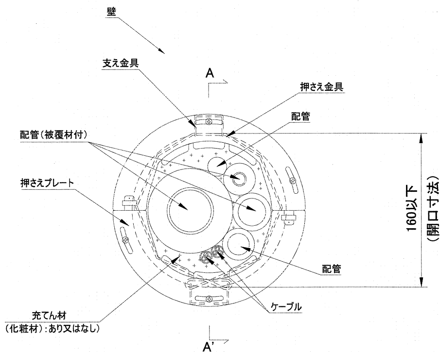
配管（被覆材付、無し）およびケーブルが混在する場合 立面図
