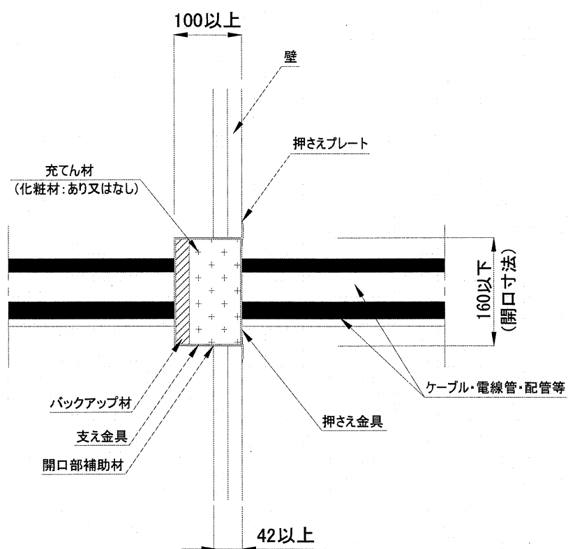
A-A' 断面図
