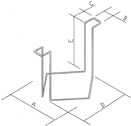
支え金具詳細図
