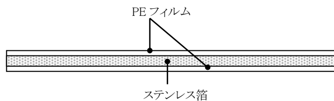
図-1 カジランシートの構造
