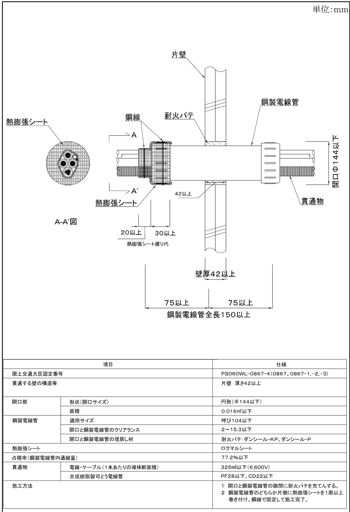
図-7 片壁(PS060WL-0867-4(PS060WL-0867、-1、-2、-3)) 標準施工図
