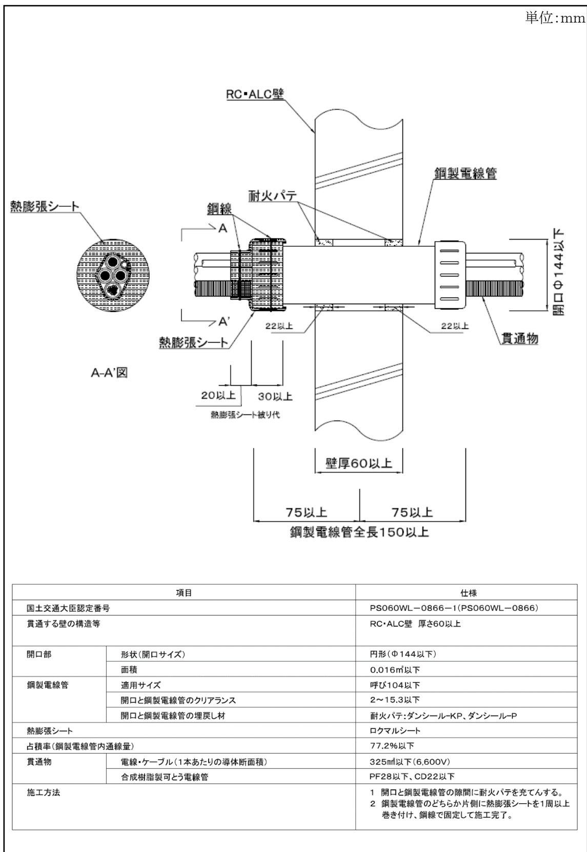
図-3 鉄筋コンクリート・ALC 壁(PS060WL-0866-1(PS060WL-0866)) 標準施工図
