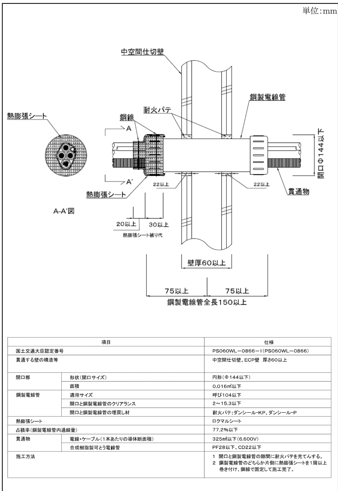
図-5 中空仕切壁(PS060WL-0866-1(PS060WL-0866)) 標準施工図
