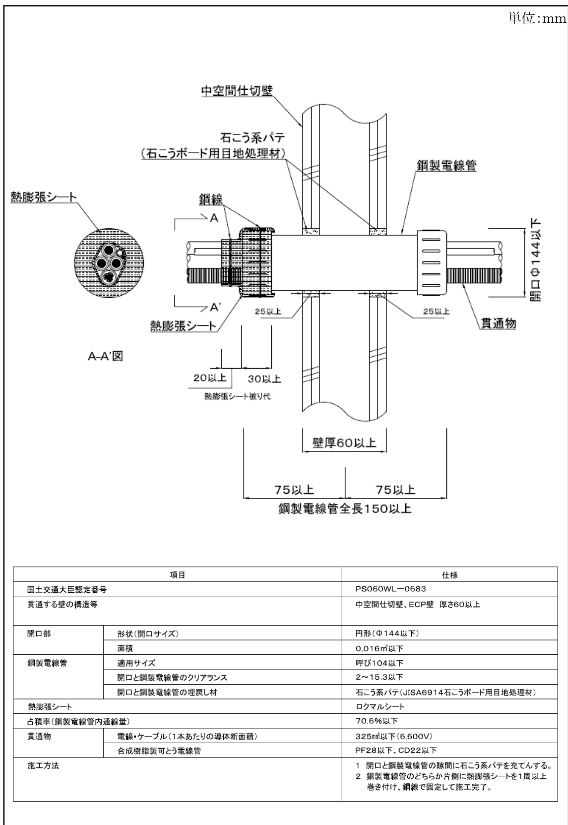
図-4 中空間仕切壁(PS060WL-0683) 標準施工図
