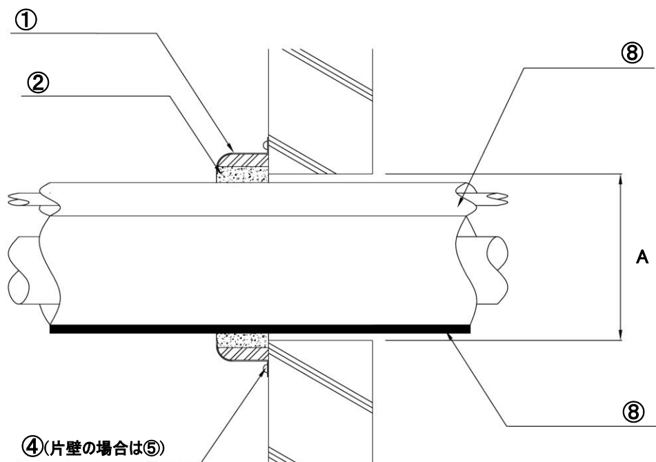
断面図
