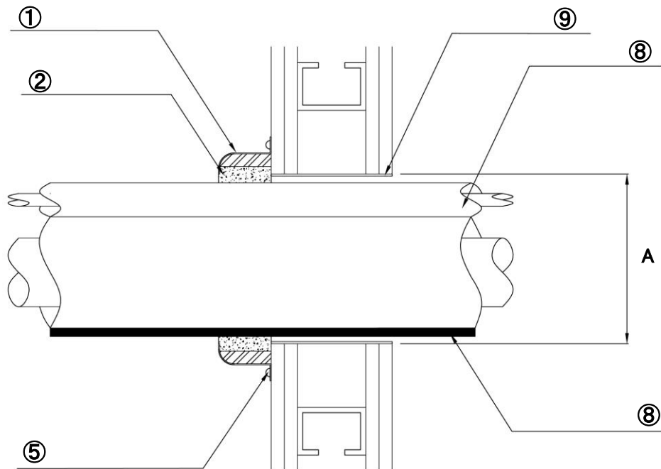
断面図
