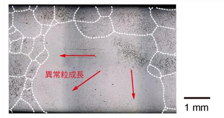
図 1: 異常粒成長により一つの結晶粒が粗大化する様子(白点線は各結晶粒の境界)
