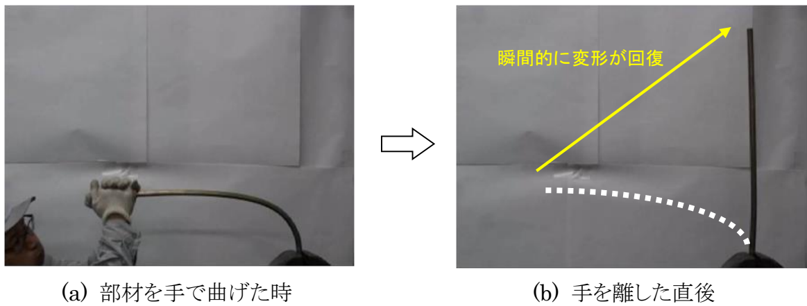
図 2: 単結晶形状記憶合金部材の変形回復の様子
