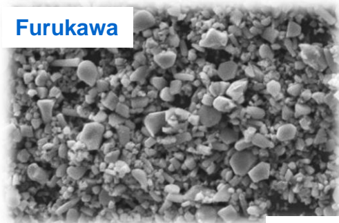
介在物の比較 (SPEED法による介在物の抽出後)
